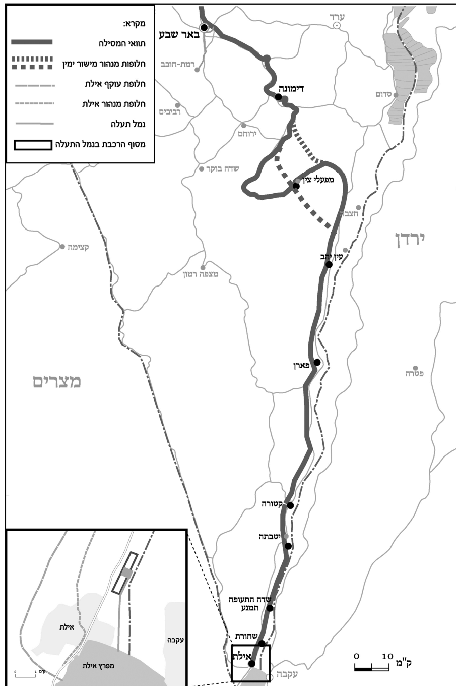
איור 1.1: תוואי המסילה לאילת - חלופות
